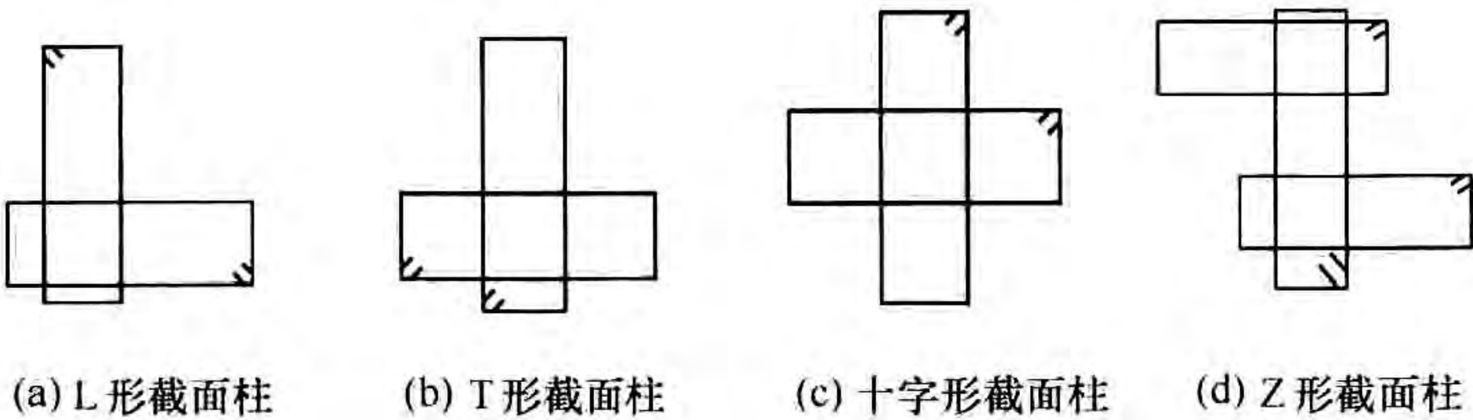
图 6.2.7 箍筋形式
