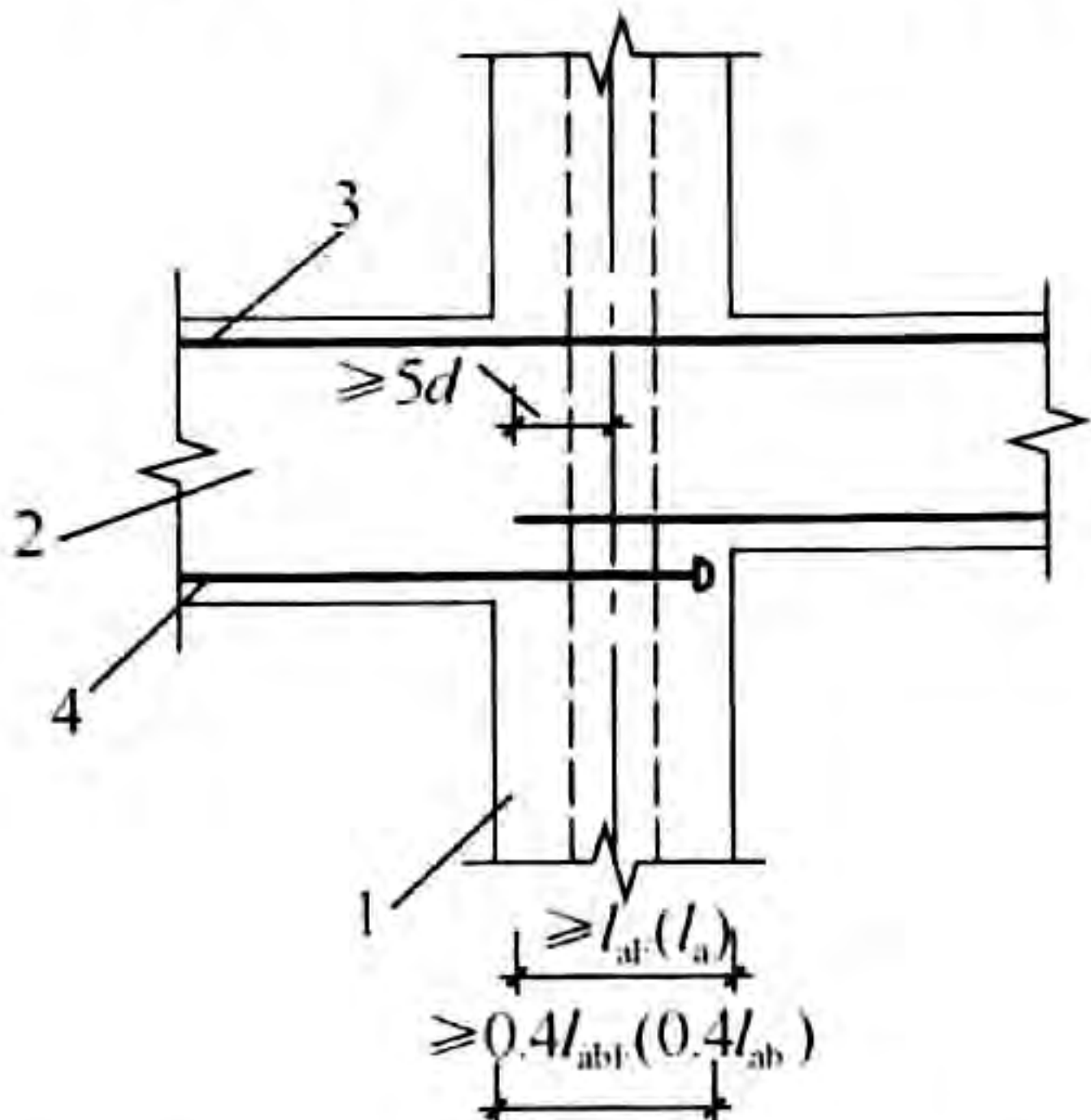
(b) 等高梁节点梁钢筋锚固板锚固
